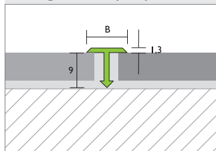
Représentation schématique / Possibilité de montage Largeur = 14 | 20 | 25 mm
