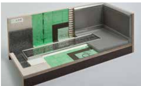
PROCHANNEL p-line avec grille design Réf.: M31469 (Dimension: 508 x 210 x 198 mm)
