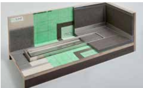
PROCHANNEL s-line avec grille à carrelage Réf.: M31468 (Dimension: 508 x 210 x 198 mm)
