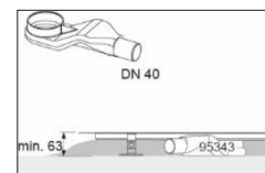
Siphon ultraplat
