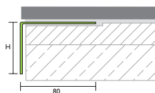
folded / avec arêtes
