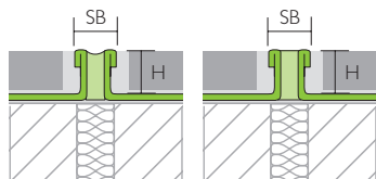
Design close to surface | Surface peu excavée
