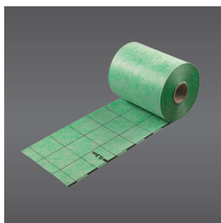
PROFOLIO 2.0 Stoßverbindungsband
