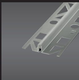
PROCONNEX Dünnbettprofile
