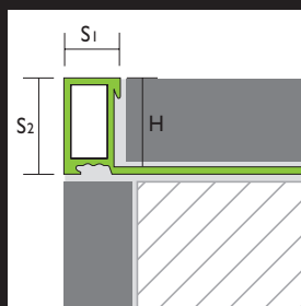
PRODECOR R
