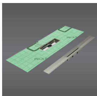
PROCHANNELd-line Duschprofil
