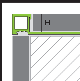
PRODECOR Q
