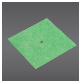
PROFOLIO 2.0 Dichtbändecken
