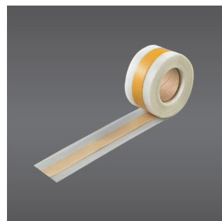
PROBAND Stoßverbindungsband
