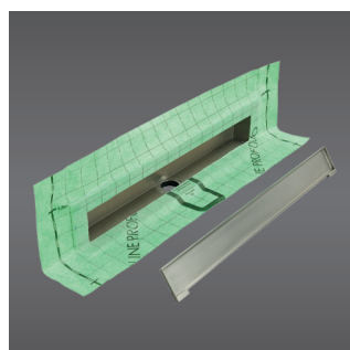
PROCHANNELw-line Wandablauf
