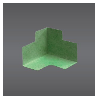
PROFOLIO 2.0 Dichtmanschetten
