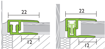
with height adjustment elements | avec pièces d'élévation
