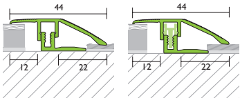
with height adjustment elements | avec pièces d'élévation
