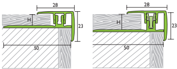
with height adjustment elements | avec pièces d'élévation
